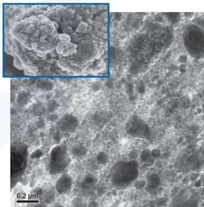
Рис. В: Электронная микрофотография (TEM) универсального наногибридного композитного материала Filtek™ Z550 (увеличение в 11 000 раз). Электронная микрофотография нанокластера в составе универсального наногибридного композитного материала Filtek™ Z550 (увеличение в 100 000 раз).
