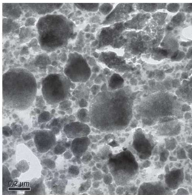
Рис. А: Электронная микрофотография (TEM) универсального микрогибридного композитного материала Filtek™ Z250 (увеличение в 11 000 раз).
