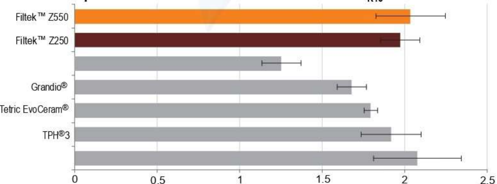
Прочность на изгиб K1c
