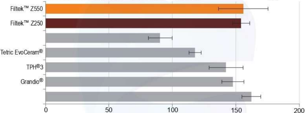
Стойкость к распространению трещин MPa
