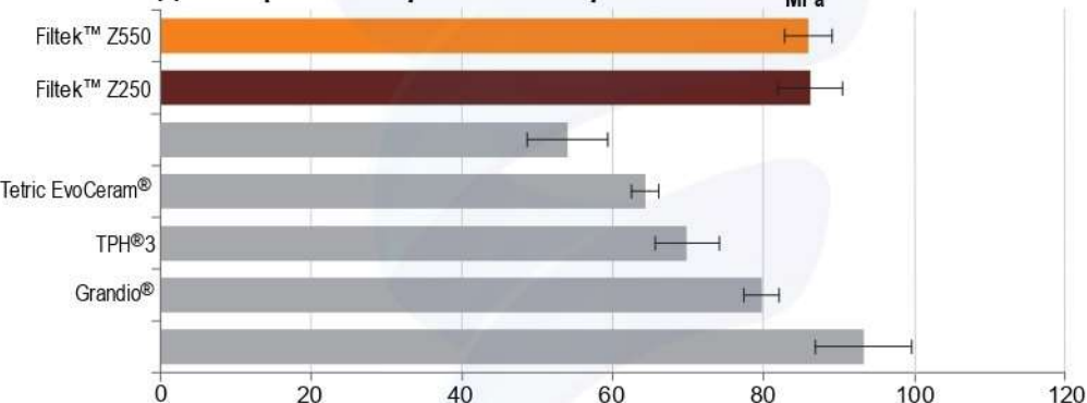
Диаметральная прочность на растяжение MPa
